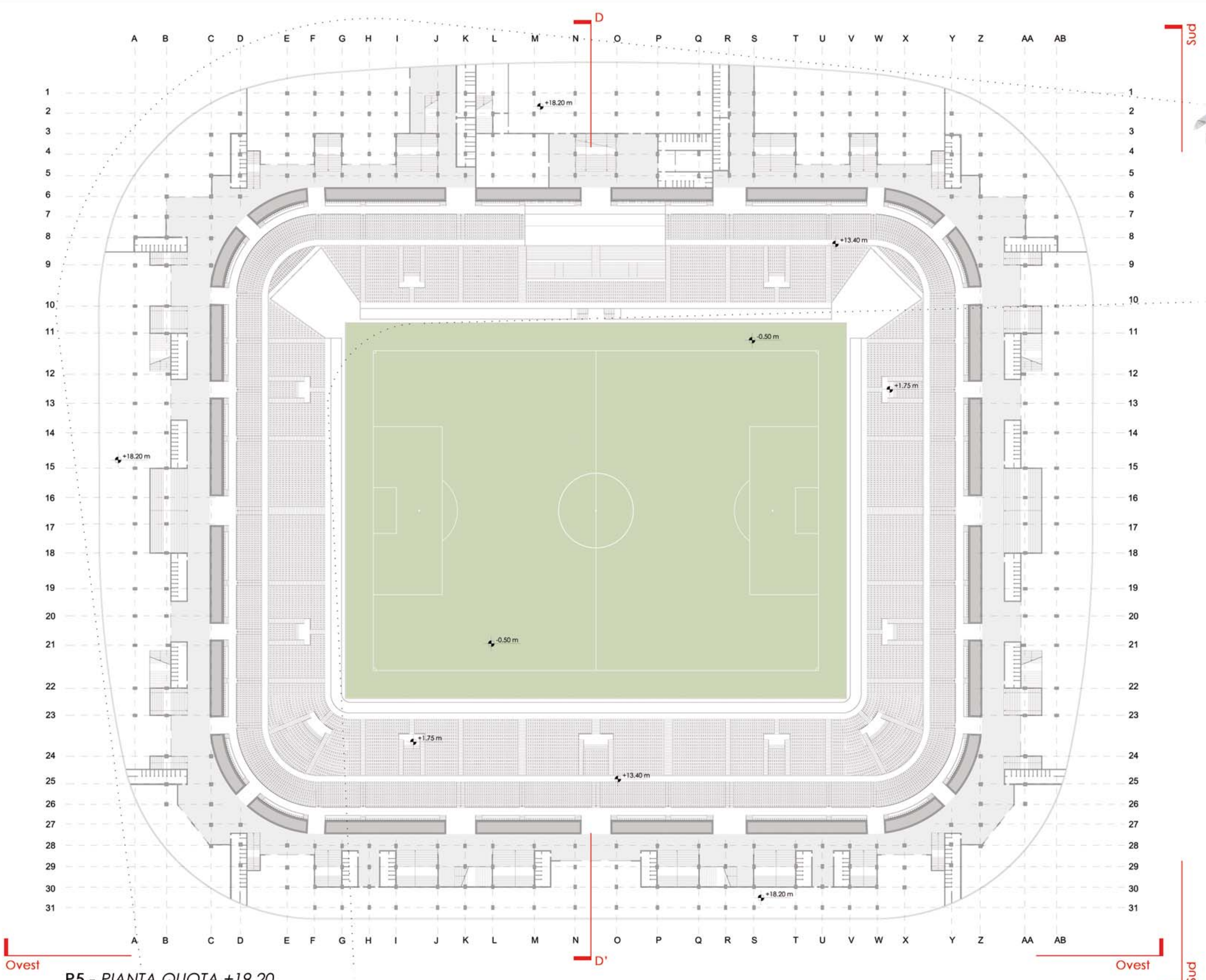
P5 - PIANTA QUOTA +19.20 Rapp. 1:500
