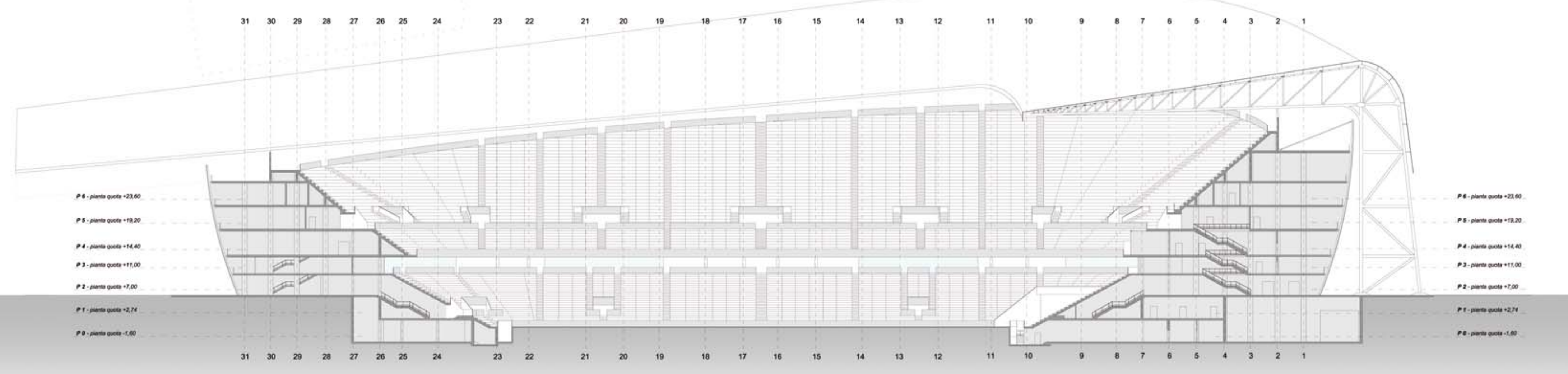
SEZIONE D-D' Rapp. 1:500
