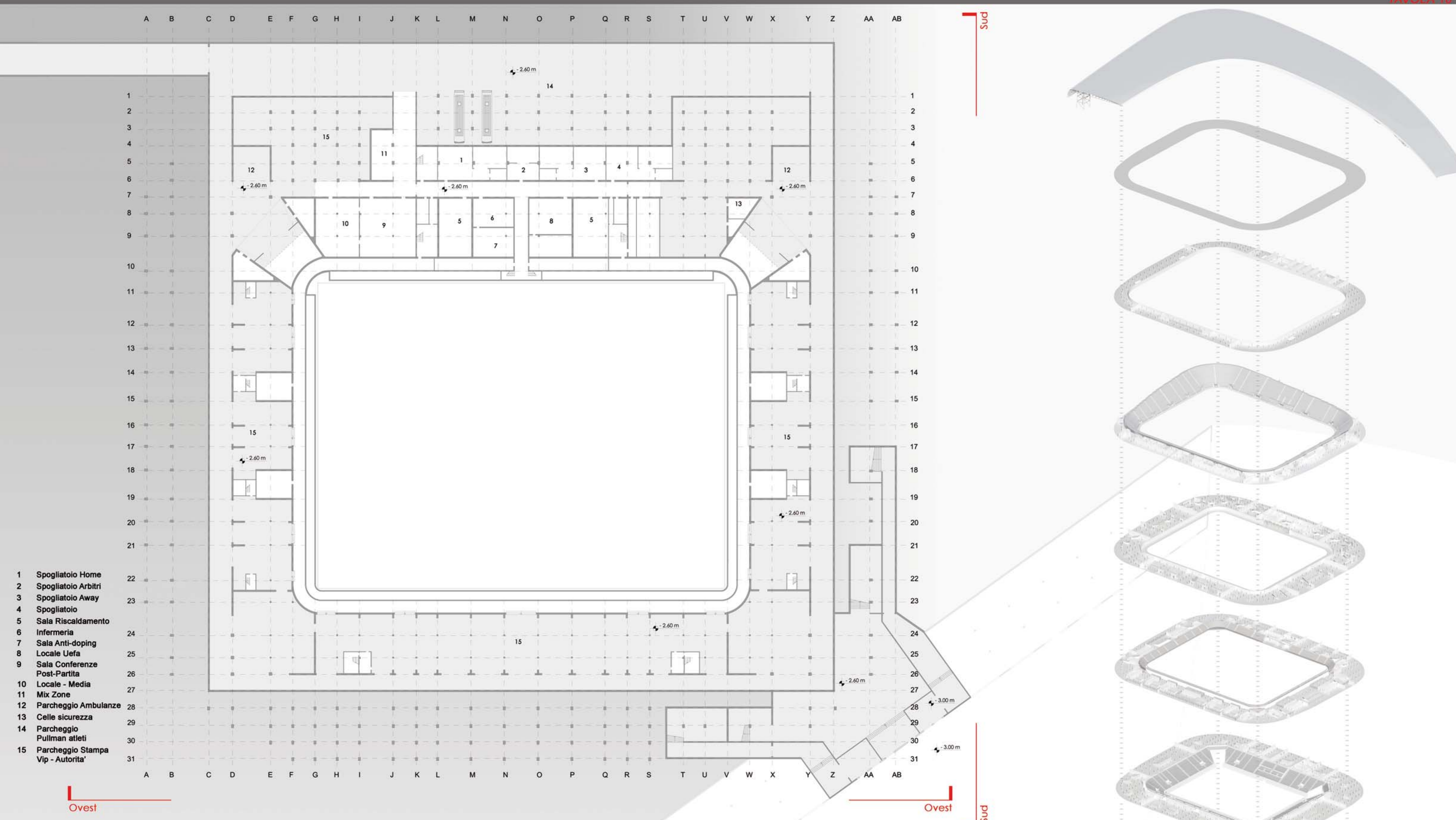
P0 - Pianta Quota -1.60 Rapp. 1:500
