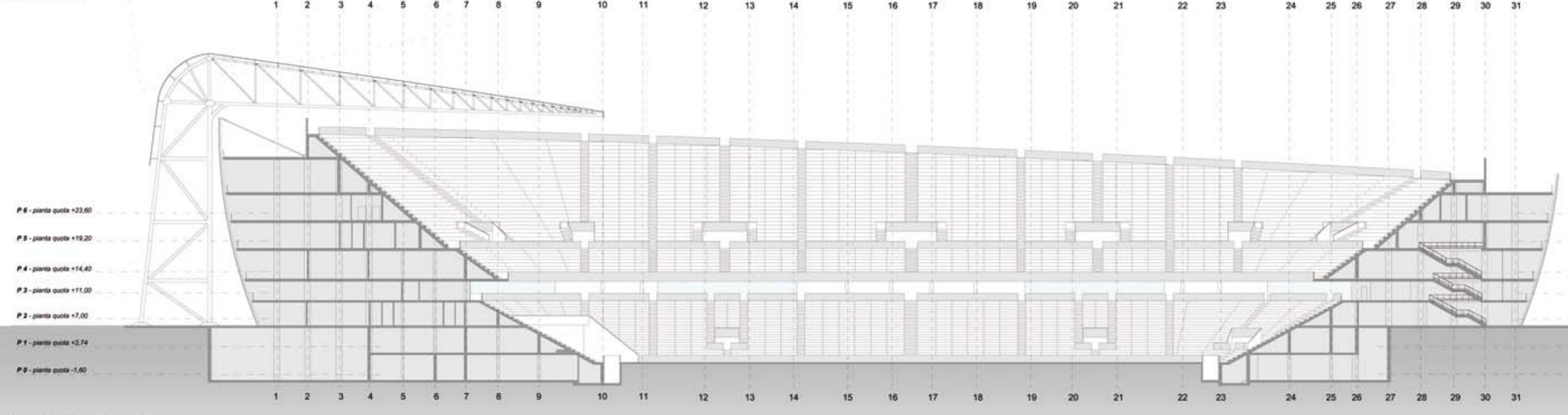
SEZIONE C-C' Rapp. 1:500
