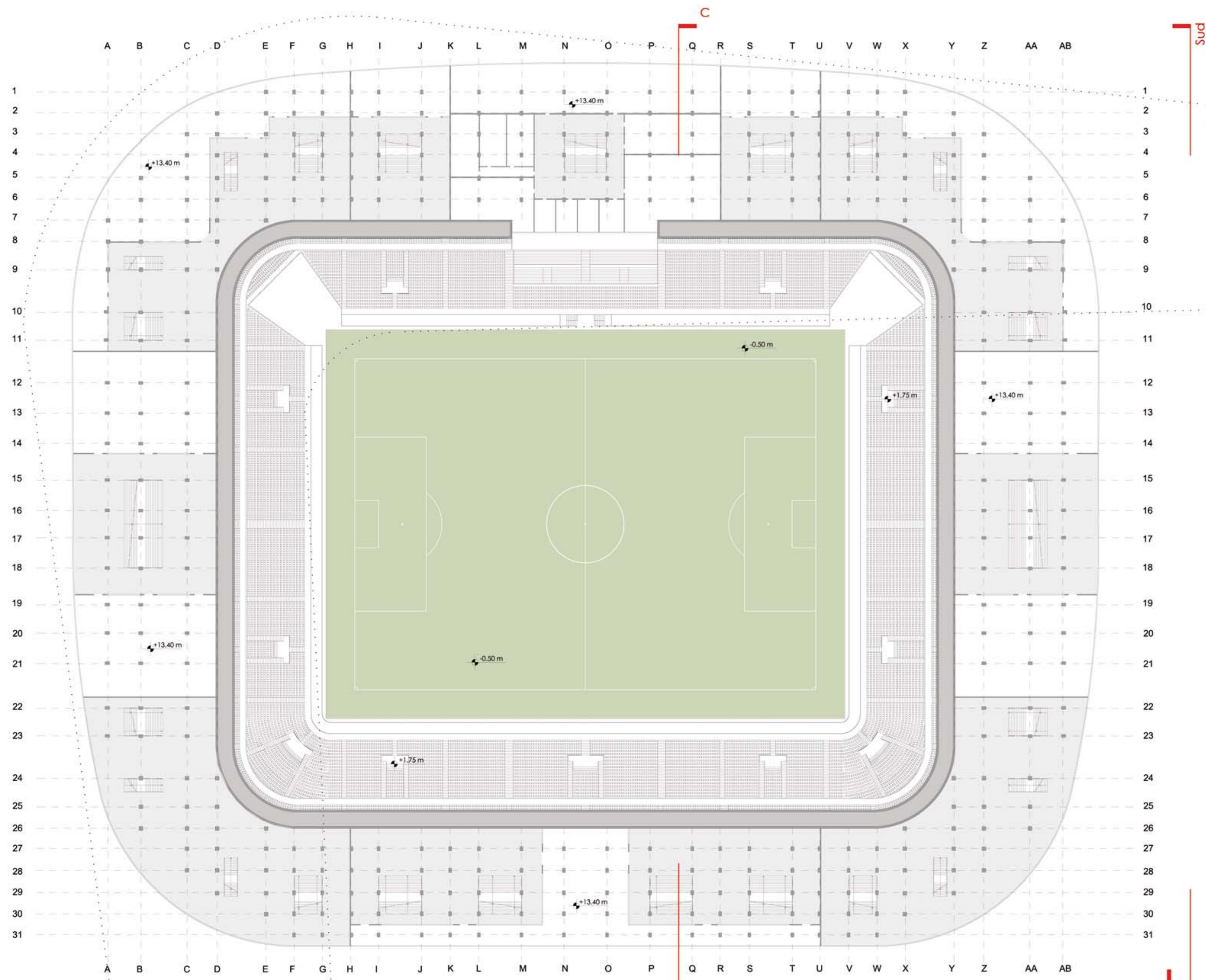
P4 - PIANTA QUOTA +14.40 Rapp. 1:500
